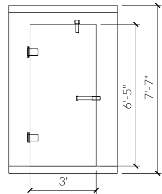
36" WIDE DOOR
